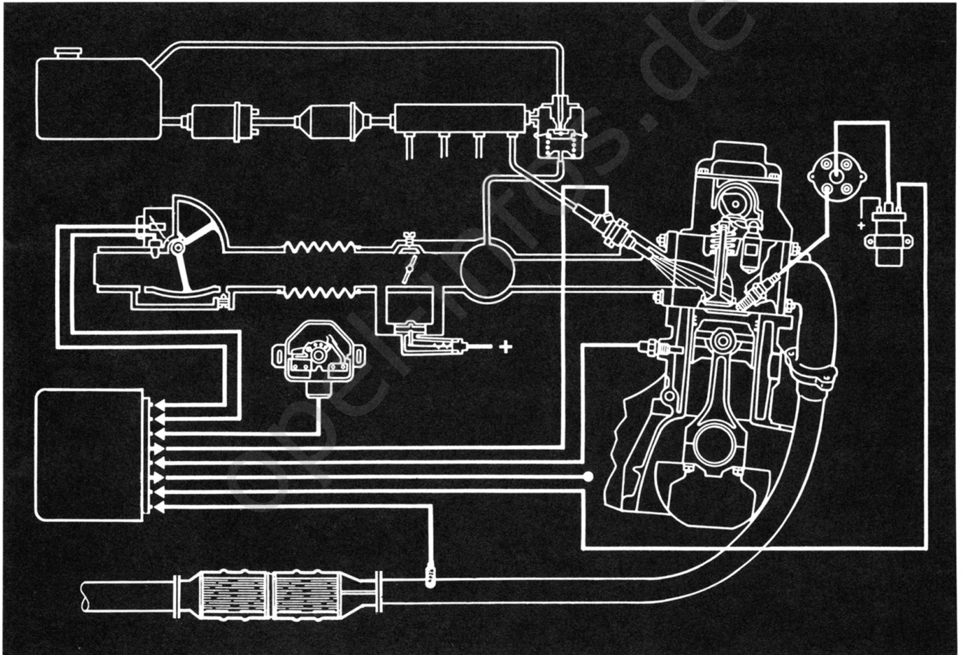
Funktionsschema lambda-geregelter Dreibege-Katalysator
